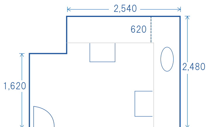
メイクルーム 2 H=2,480
